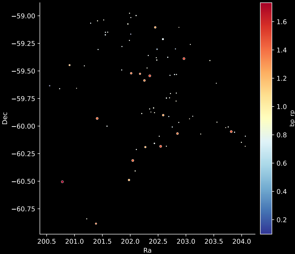
GALAH DR4 Field: [7427] Stars: 81
