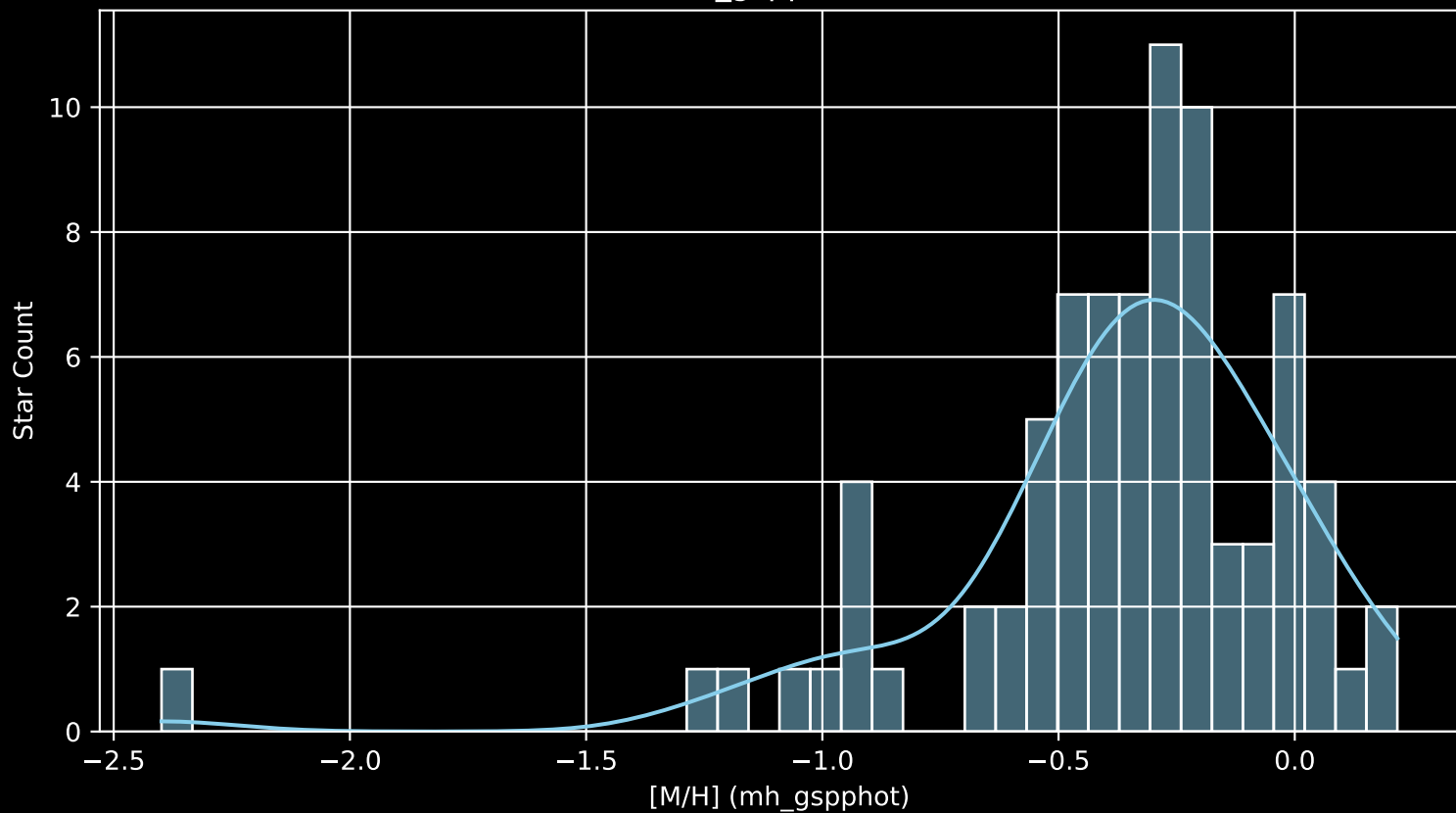
GALAH DR4 Field: [7427] [M/H] (mh_gspphot) (n= 81)
