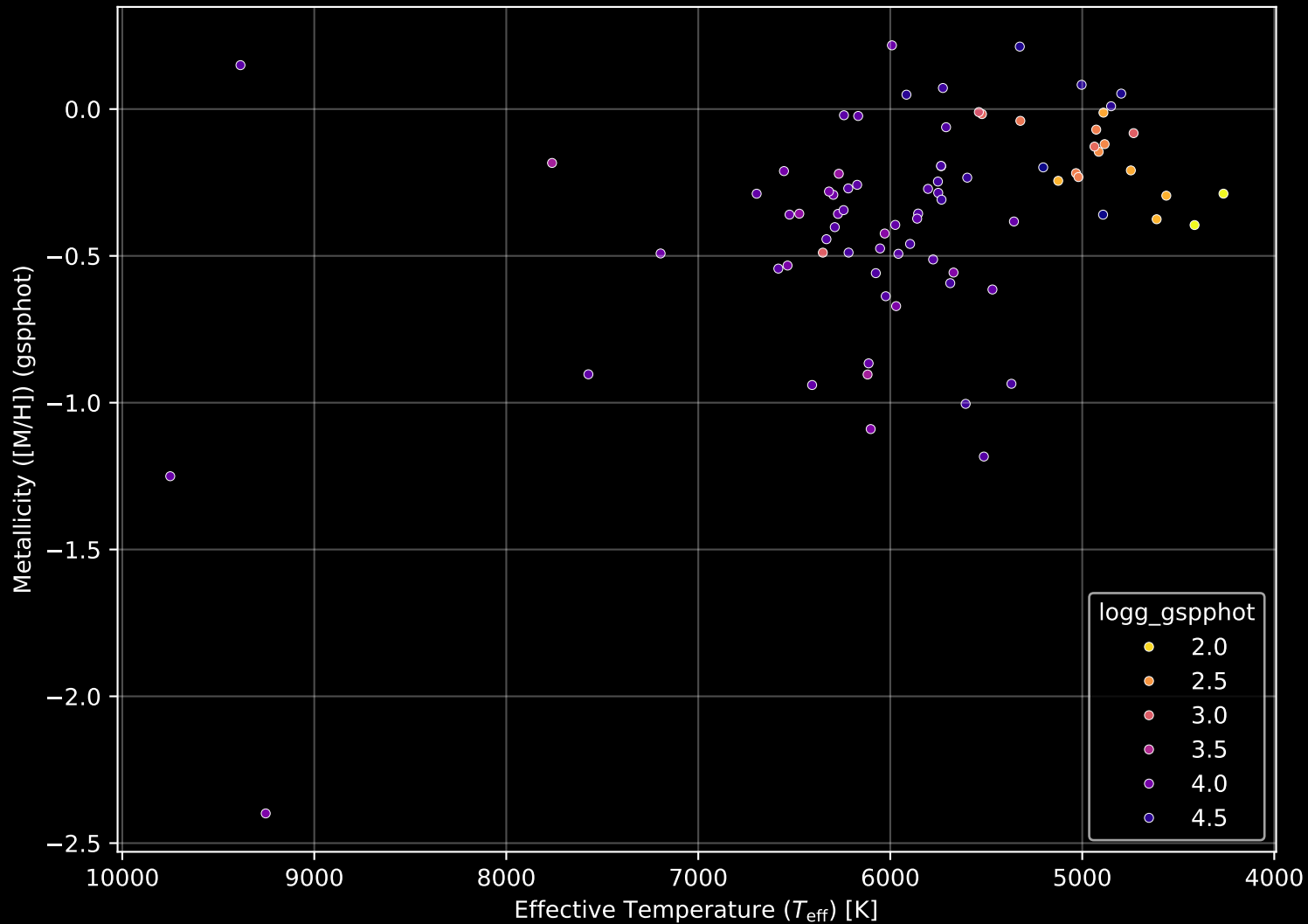
GALAH DR4 Field: [7427] Stellar Population Parameters (n= 81)
