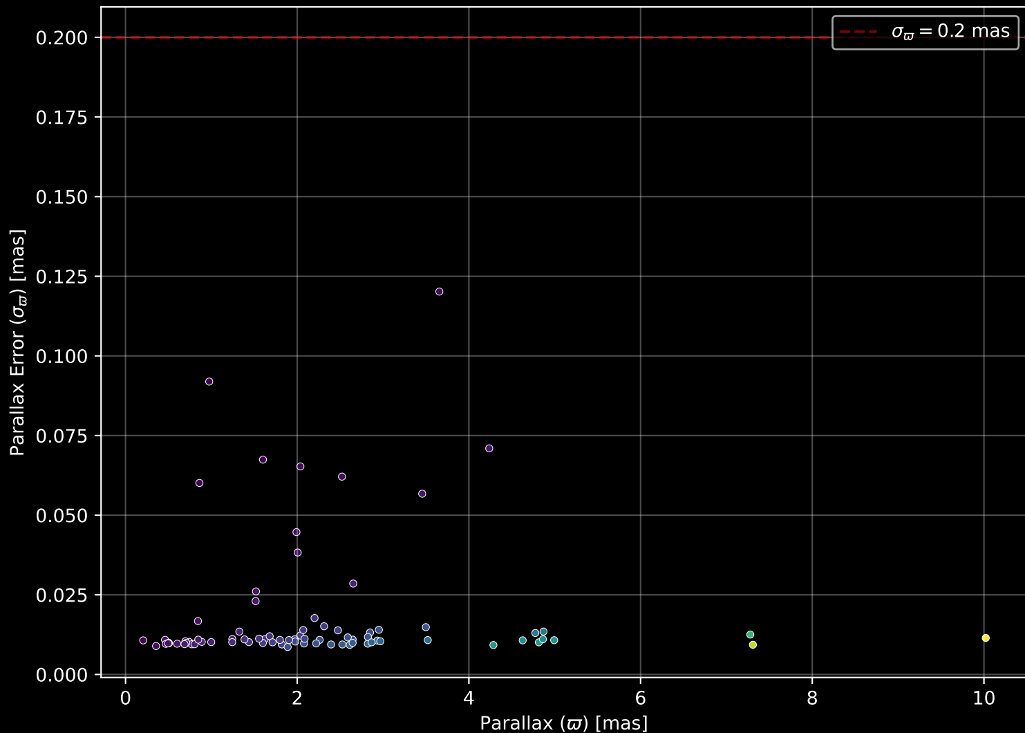
GALAH DR4 Field: [7427] Parallax Quality (n= 81)
